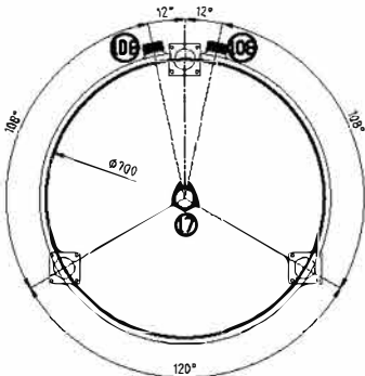
Untenansicht
